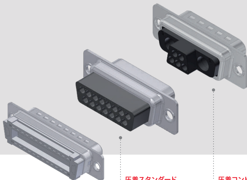
IDC (フラットケーブル) プレスコンタクト AWG28-26
